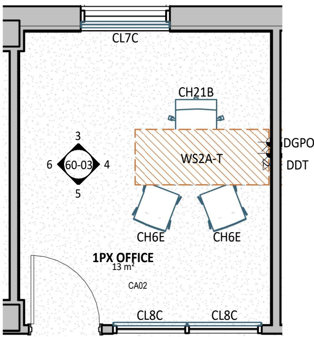
2 PLAN DETAIL 1 : 50
